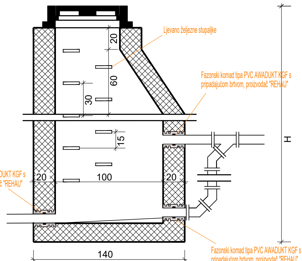
KASKADNO REVIZIJSKO OKNO
