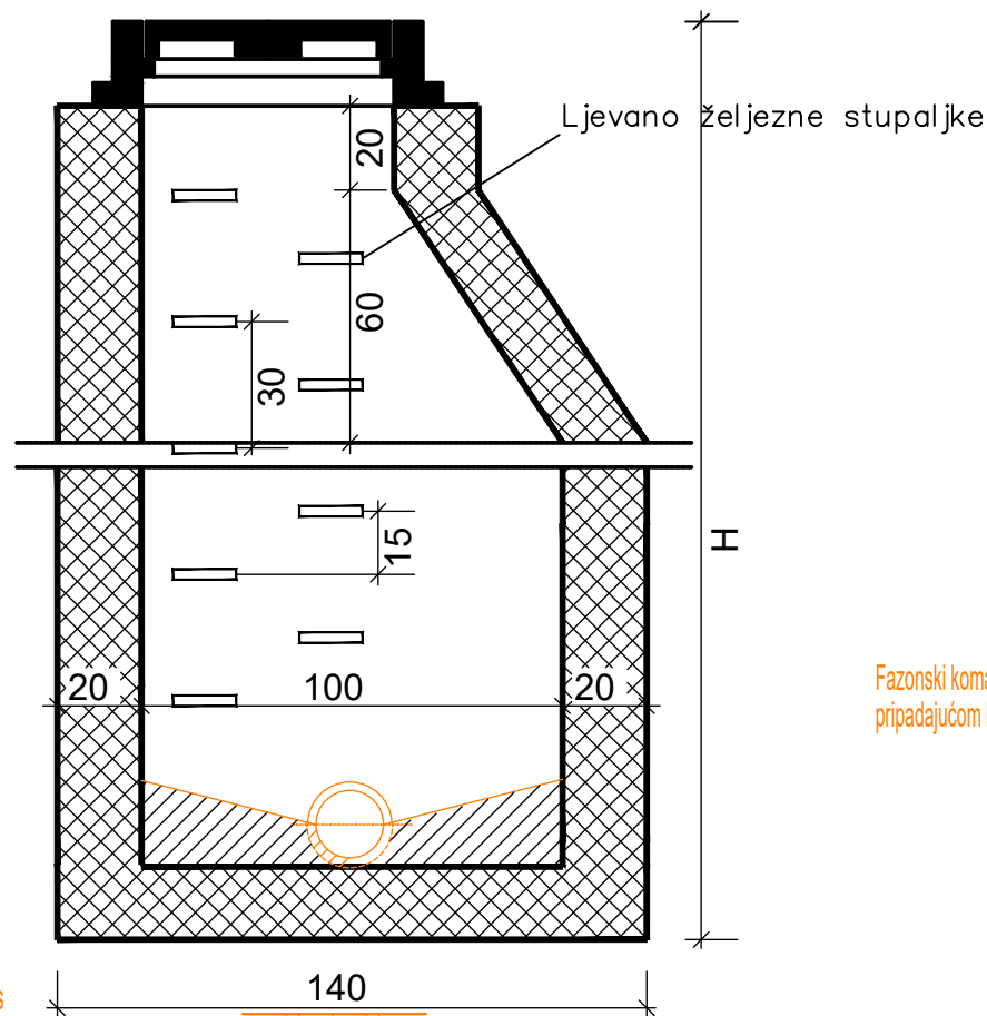
ŽLJEBNO REVIZIJSKO OKNO DUBLJE OD 120cm
